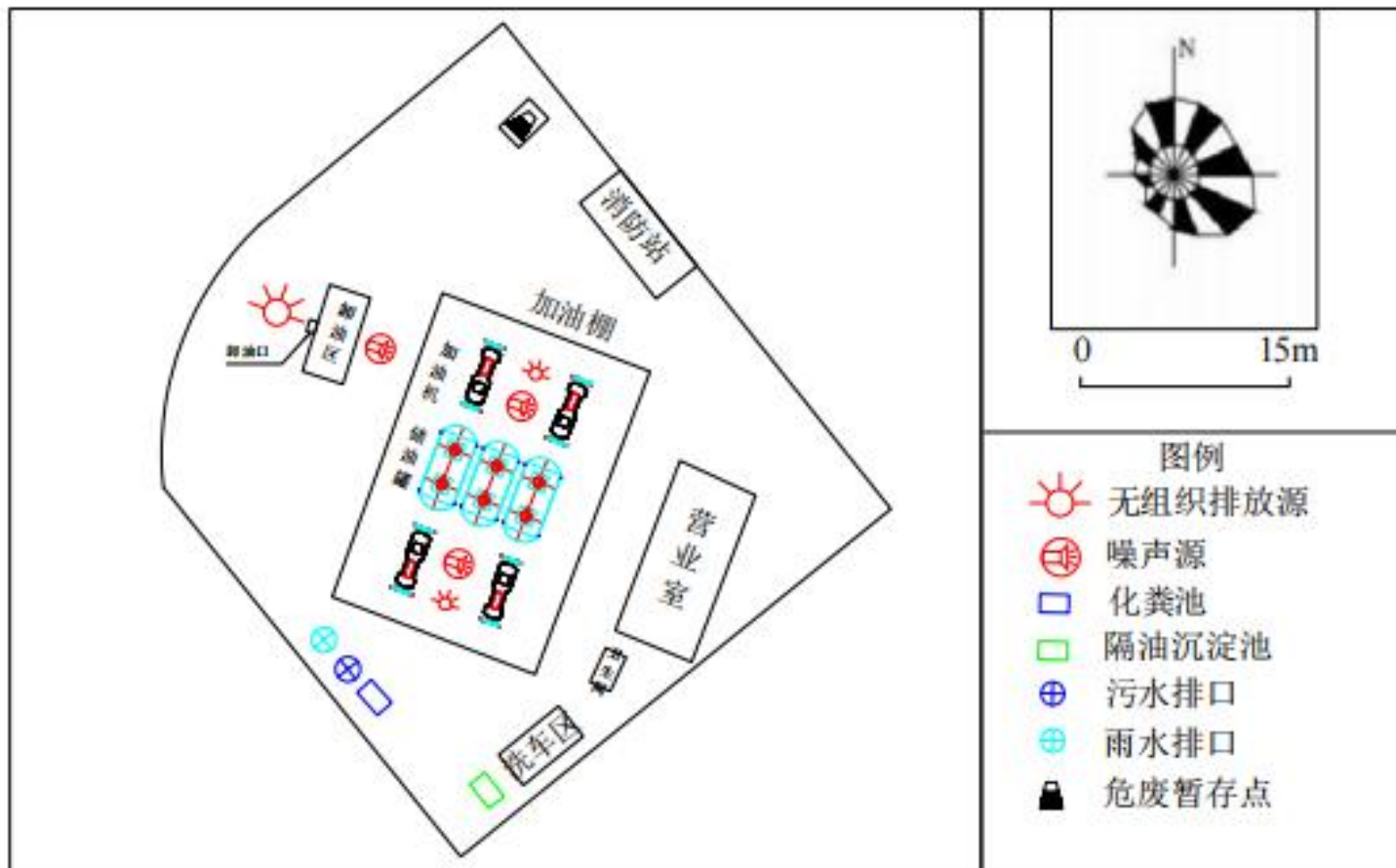
图 4-3 项目厂区平面布置图
