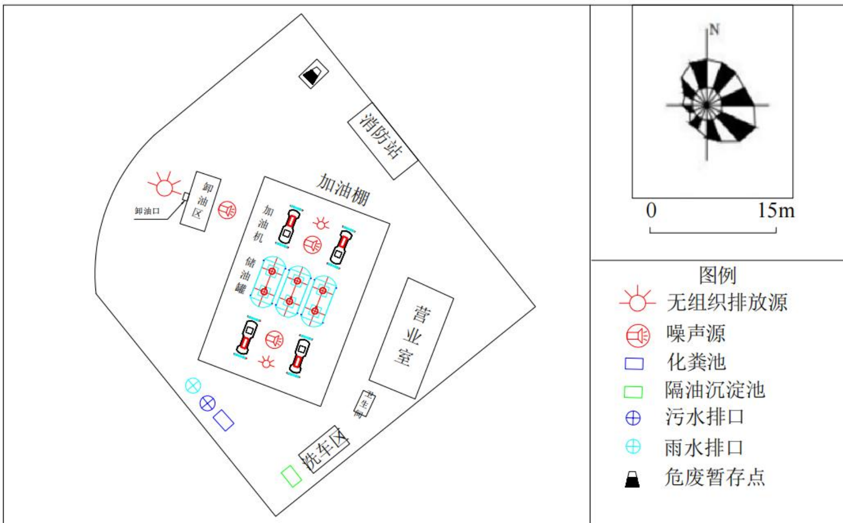
附图3 建设项目平面布置
